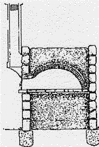
Figure 2 - Coupe du four
